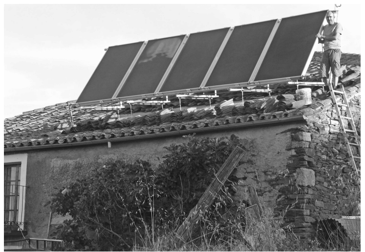
Foto: instalación solar térmica en una casa rural.
